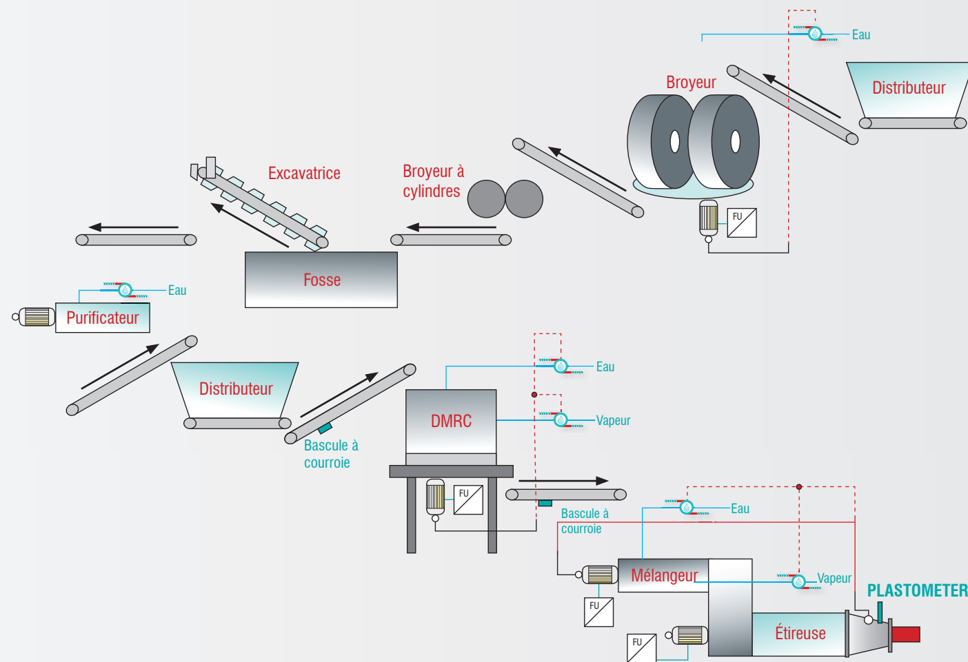
Exemple: ligne de préparation / de formage typique.
